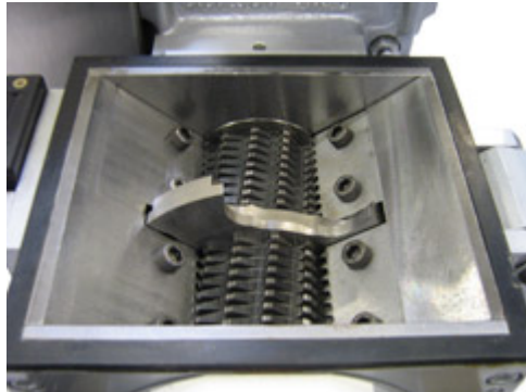
Cutting chamber Mini 1
